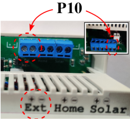
FIG 28 – Connecteur P10
