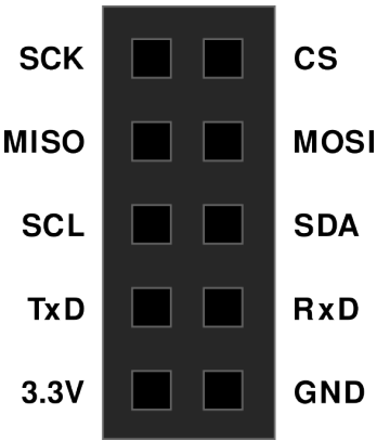
FIG 24 – Connecteur P3 - Signaux
