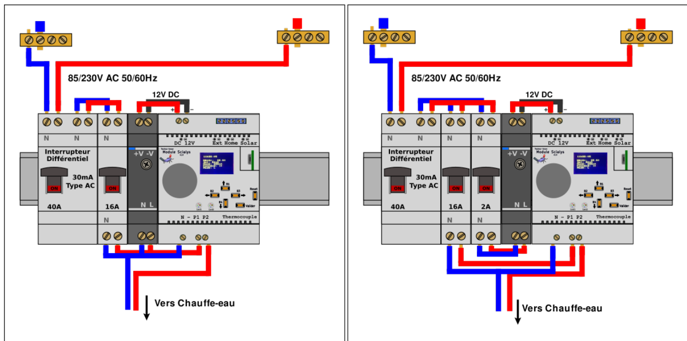
FIG 1 – Raccordement dans un tableau électrique
