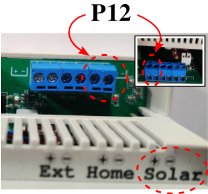
FIG 29 – Connecteur P12
