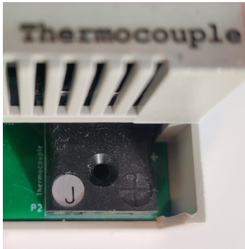
FIG 22 – Connecteur P2
