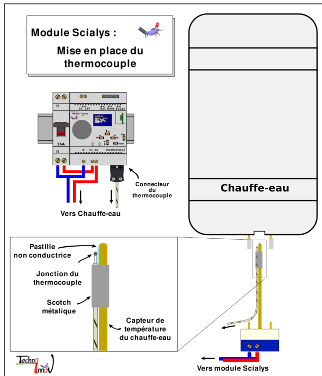
FIG 4 – Mise en place du thermocouple
