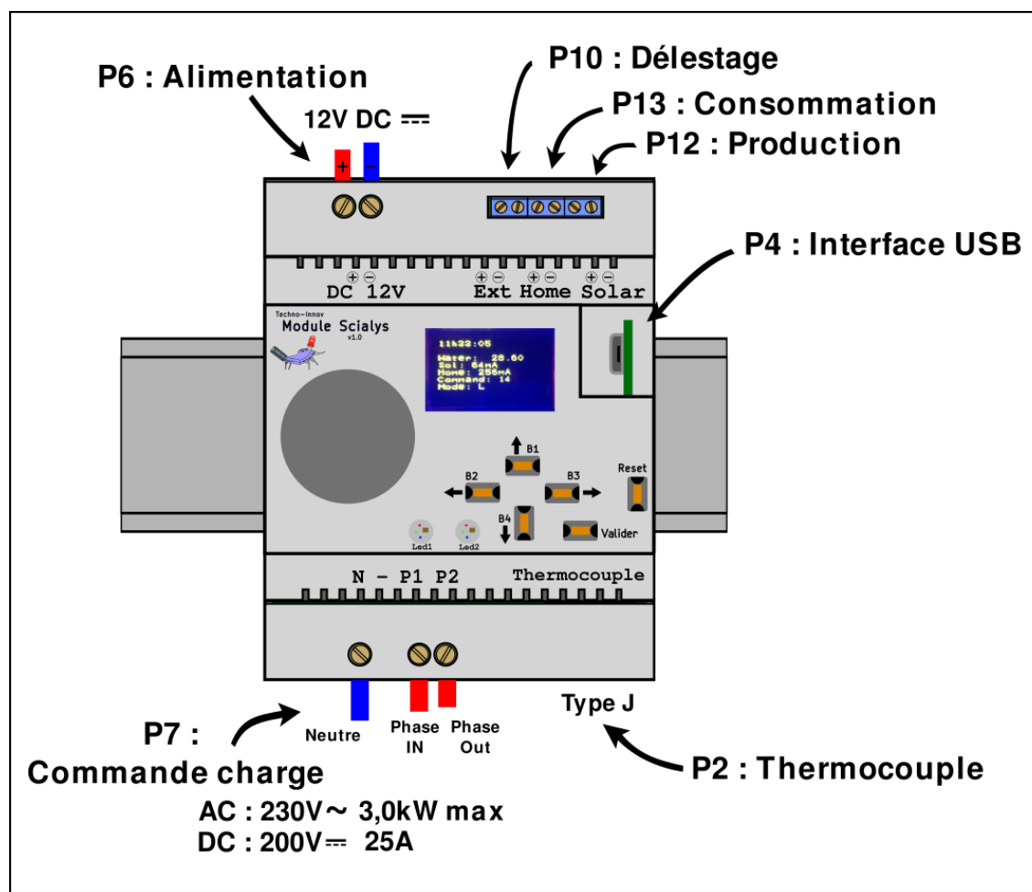
FIG 21 – Connecteurs du module Scialys
