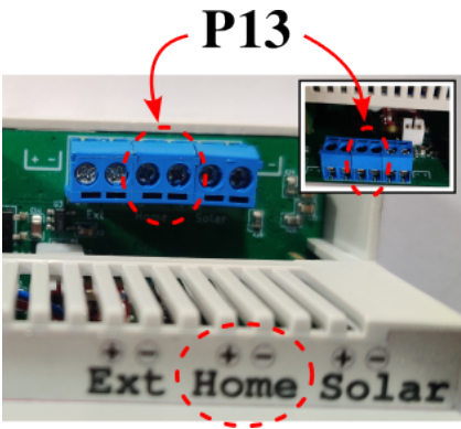
FIG 30 – Connecteur P13
