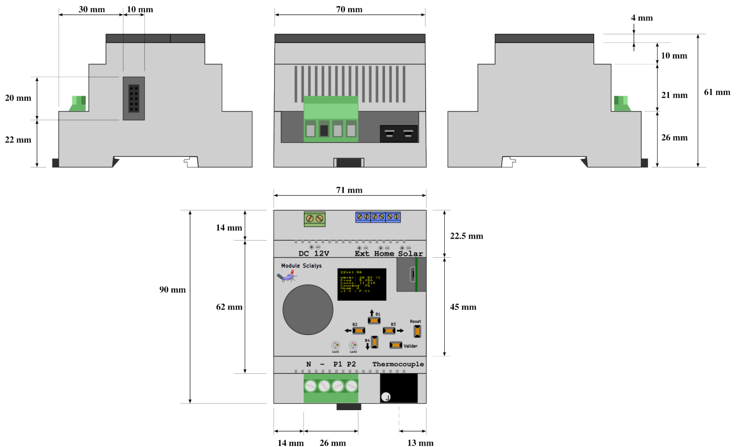
FIG 20 – Dimensions du module Scialys
