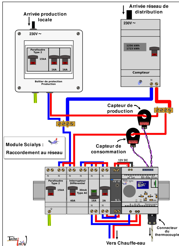
FIG 3 – Raccordement des capteurs de courant
