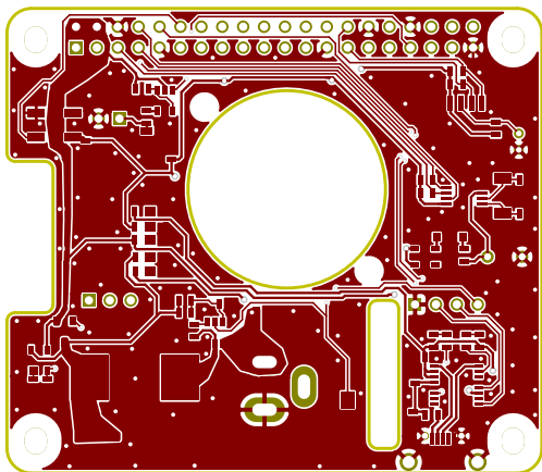
Top copper layer
