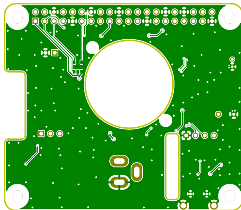
Bottom copper layer
